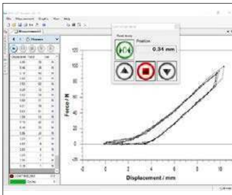
Control del banco de pruebas mediante software de ordenador SAUTER AFH
